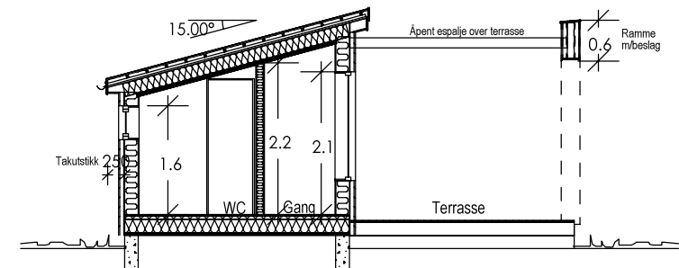
Snitt C-C
