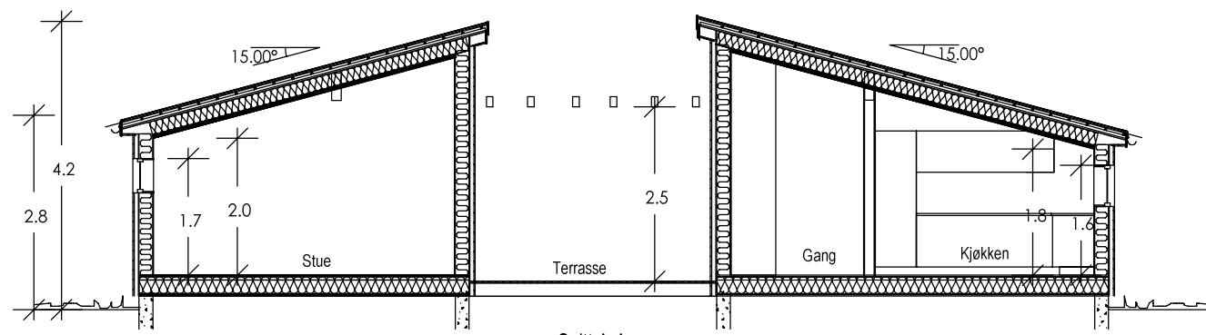
Snitt A-A
