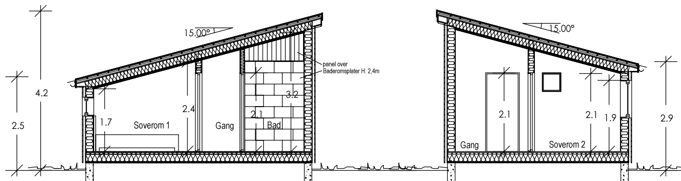
Snitt B-B
